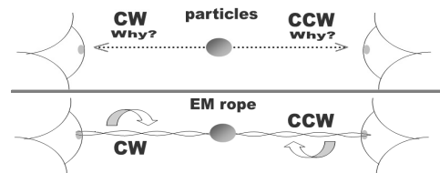
Fig. 13. EM Rope seen head on: CW spin
